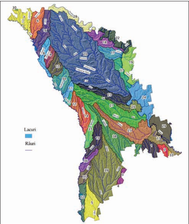
Рис. 4. Суббасейни, виділені у районах річкових басейнів на території Молдови (Centrul, 2025)
